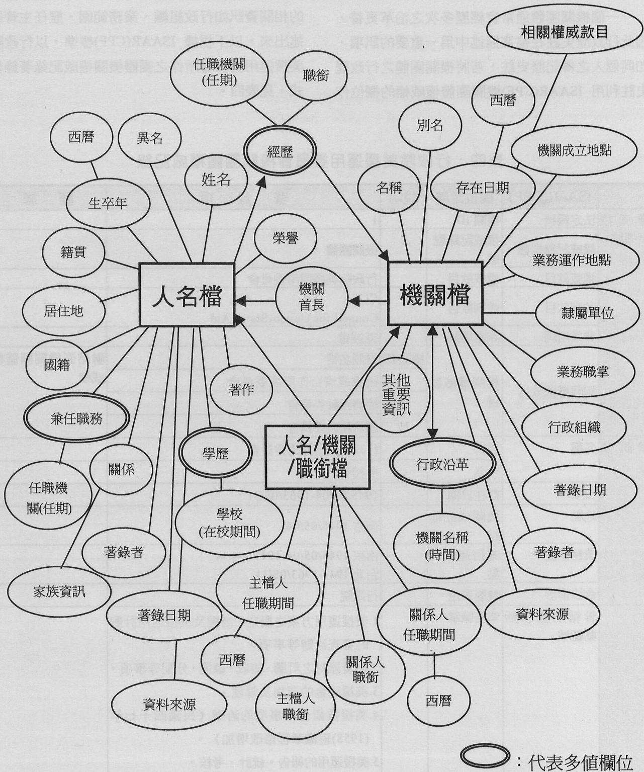
圖四：人名檔、機關檔與人名/機關/職銜檔著錄款目關聯圖
