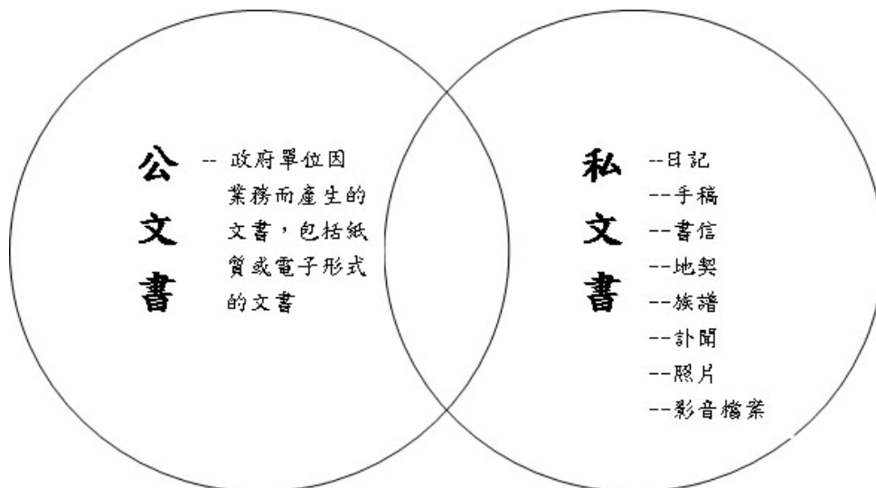
圖 1 廣義的檔案
