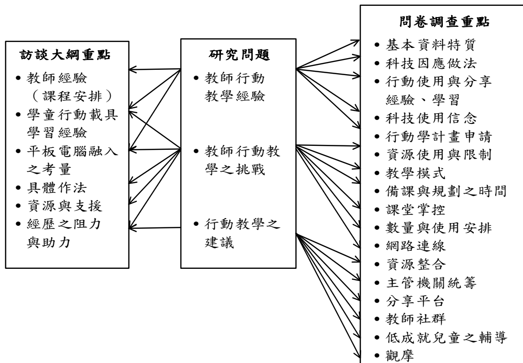
圖 1 研究之架構
